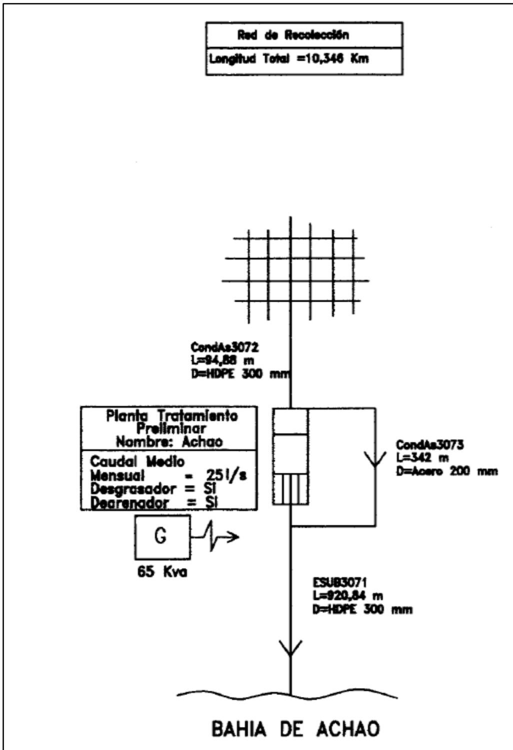
Figura 5. Esquema unilineal del Sistema de Alcantarillado de Achao.
