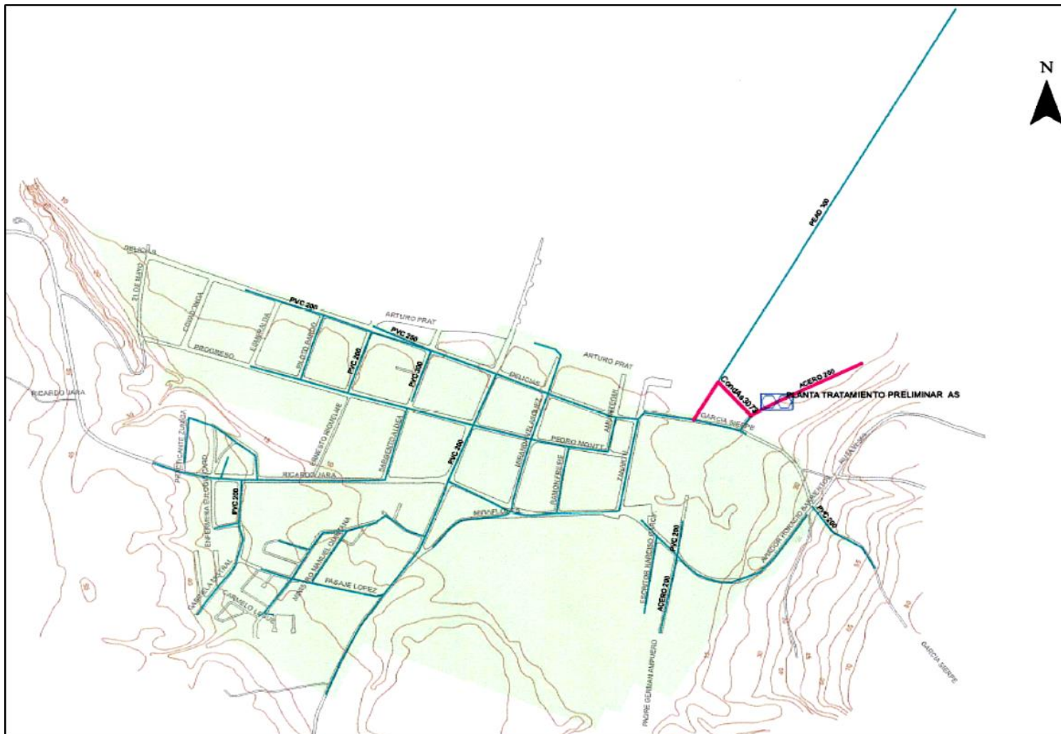
Figura 6. Esquema general de infraestructura sanitaria de alcantarillado en Achao.
