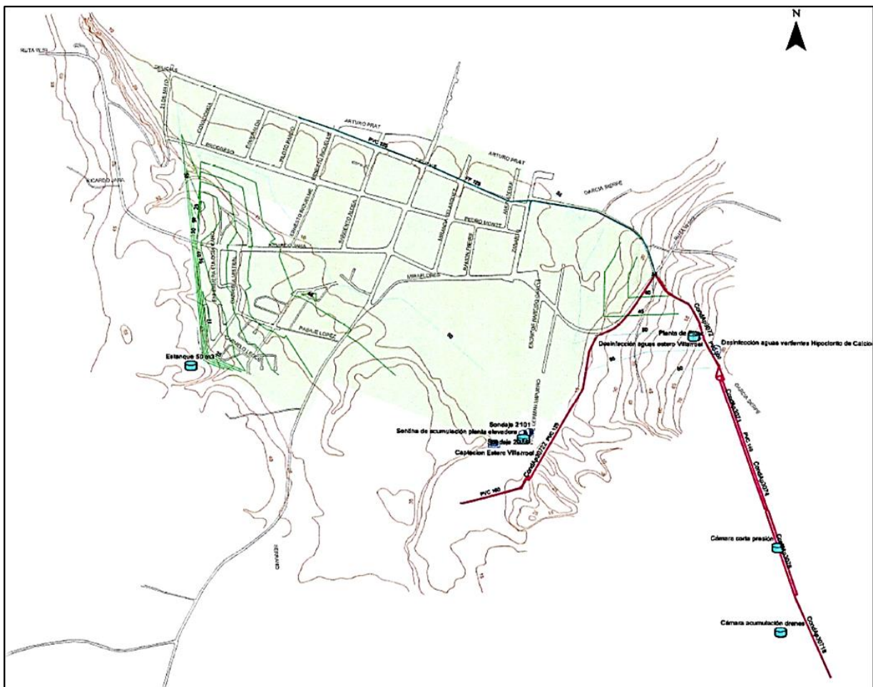
Figura 3. Infraestructura Principal de Agua Potable en Achao
