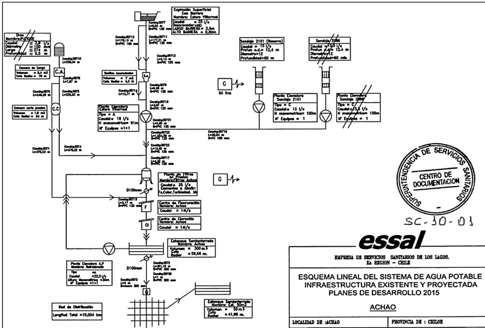
Figura 2. Esquema del Sistema de Agua Potable de Achao.
